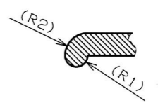
△ C-C'部詳細 (3:1)
