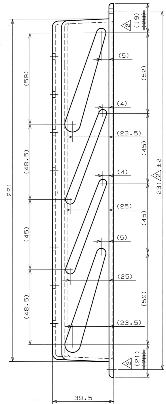
△ C-C'部詳細 (3:1)
