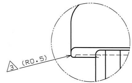
E部詳細 (3:1)
