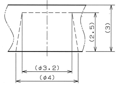
△ B部詳細 (10:1)
